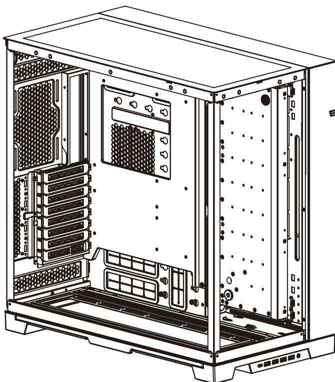
安装于机壳
